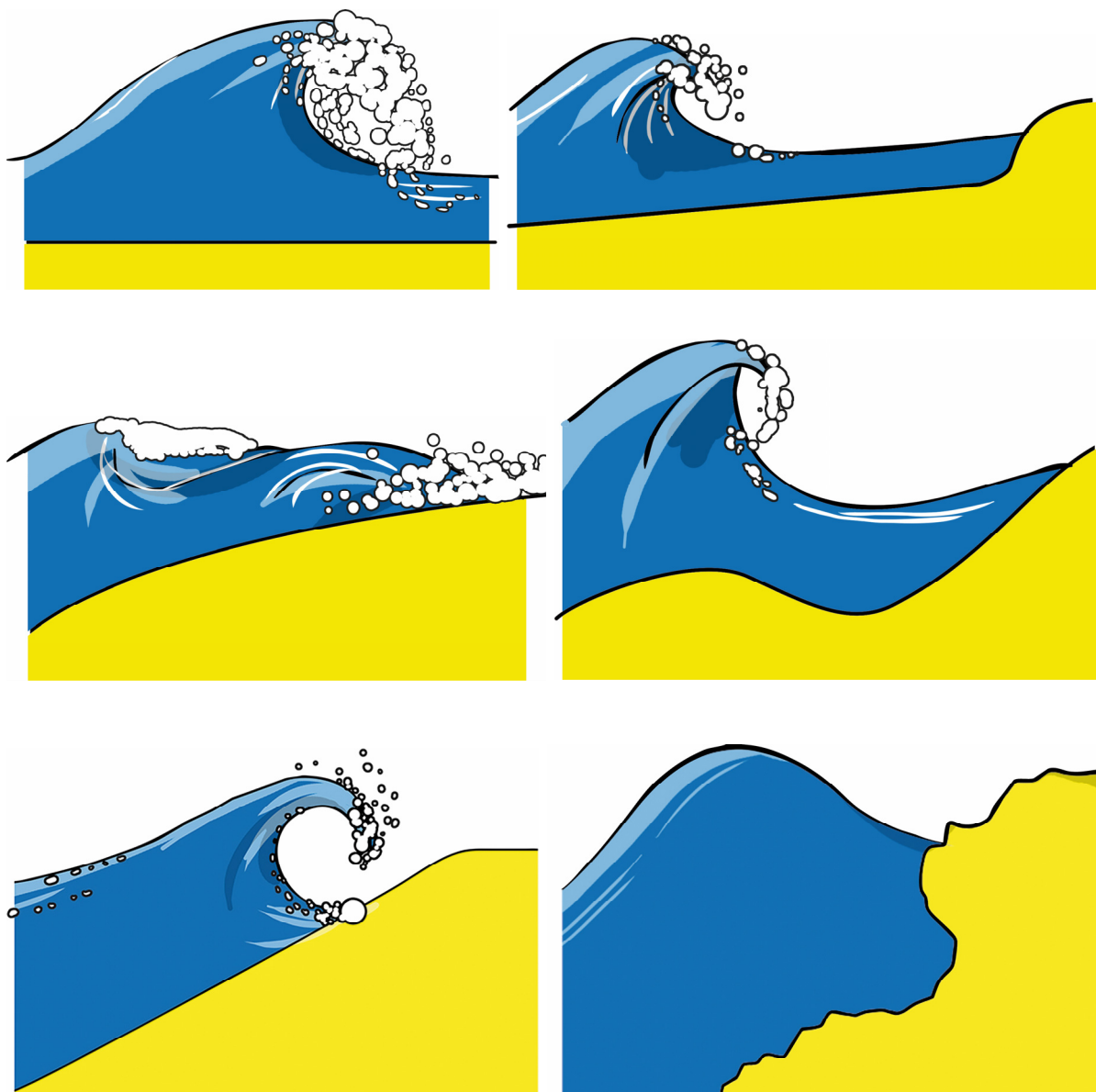
Beispiele für Wellenformen in Abhängigkeit von verschiedenen Uferformen
