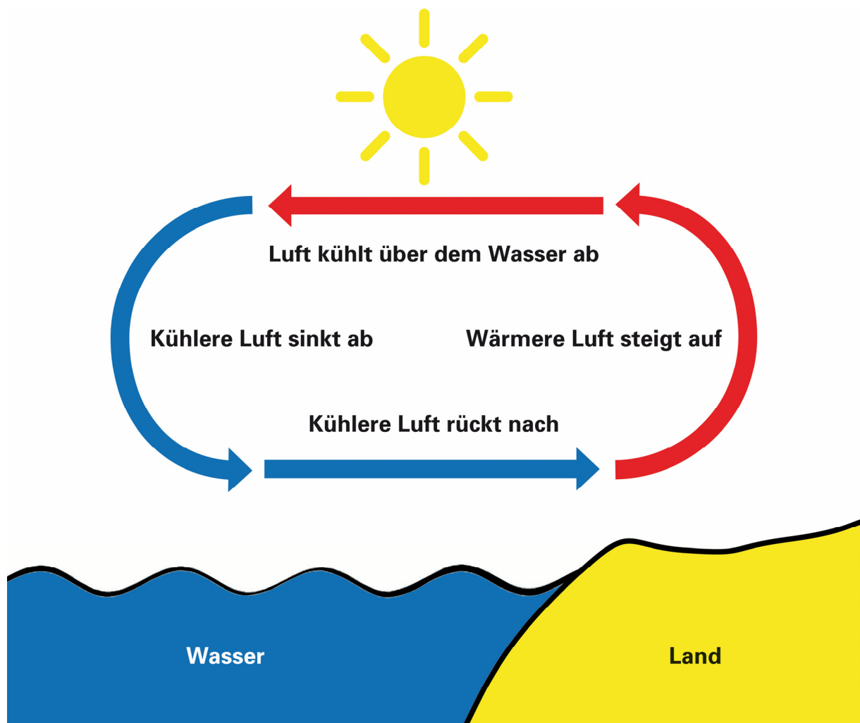
Abbildung: Entstehung von Küstenwind
