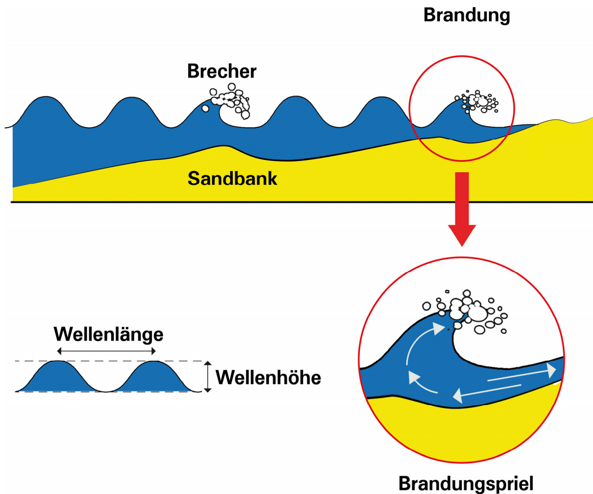
Abbildungen: Entstehung von Brandung und Begriffsdefinitionen
