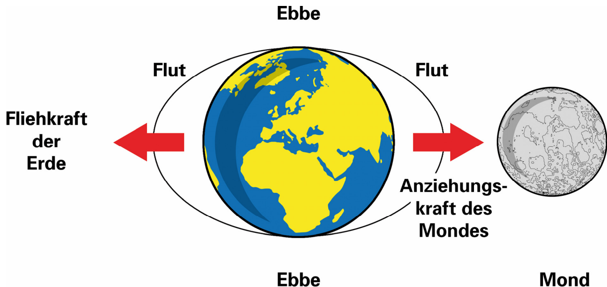
Abbildung: Entstehung von Ebbe und Flut
