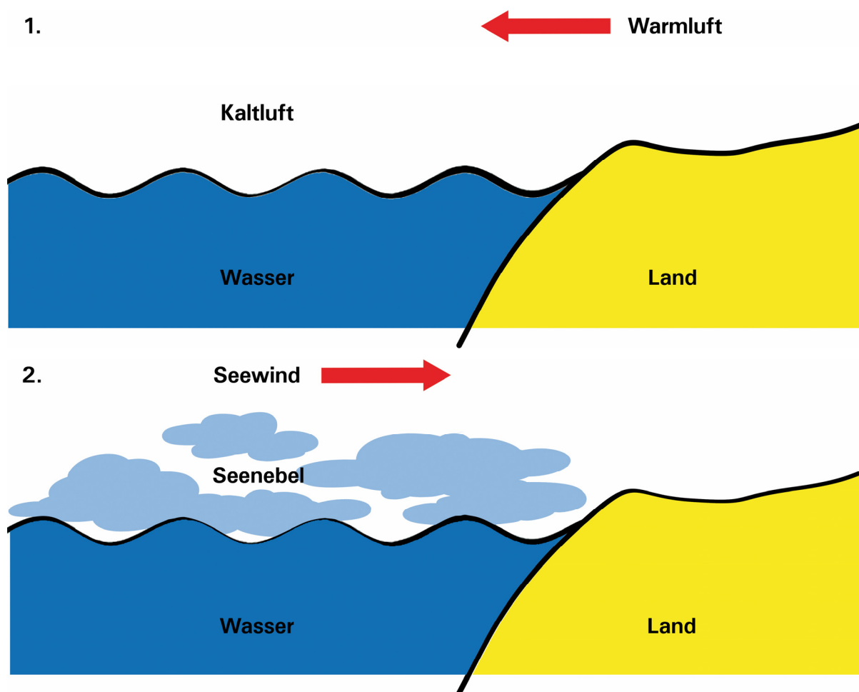
Abbildungen: Entstehung von Seenebel
